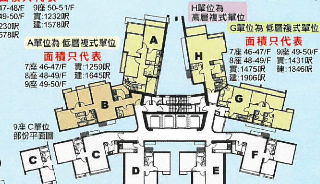
平面圖代表 BLOCK 7,8,9 座 46/F, 8座 48/F, 9座 49/F (A,G,H單位為複式單位)
