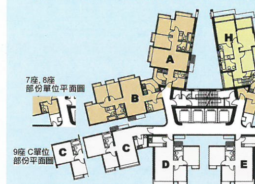
平面圖代表 BLOCK 7,8 7座 5-43/F, 8座 5-46/F
